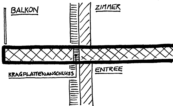
SYSTEMSCHNITT
