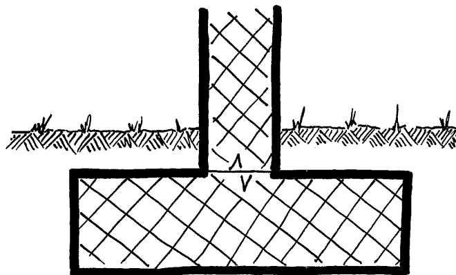
SYSTEMSCHNITT EINZELFUNDAMENT
