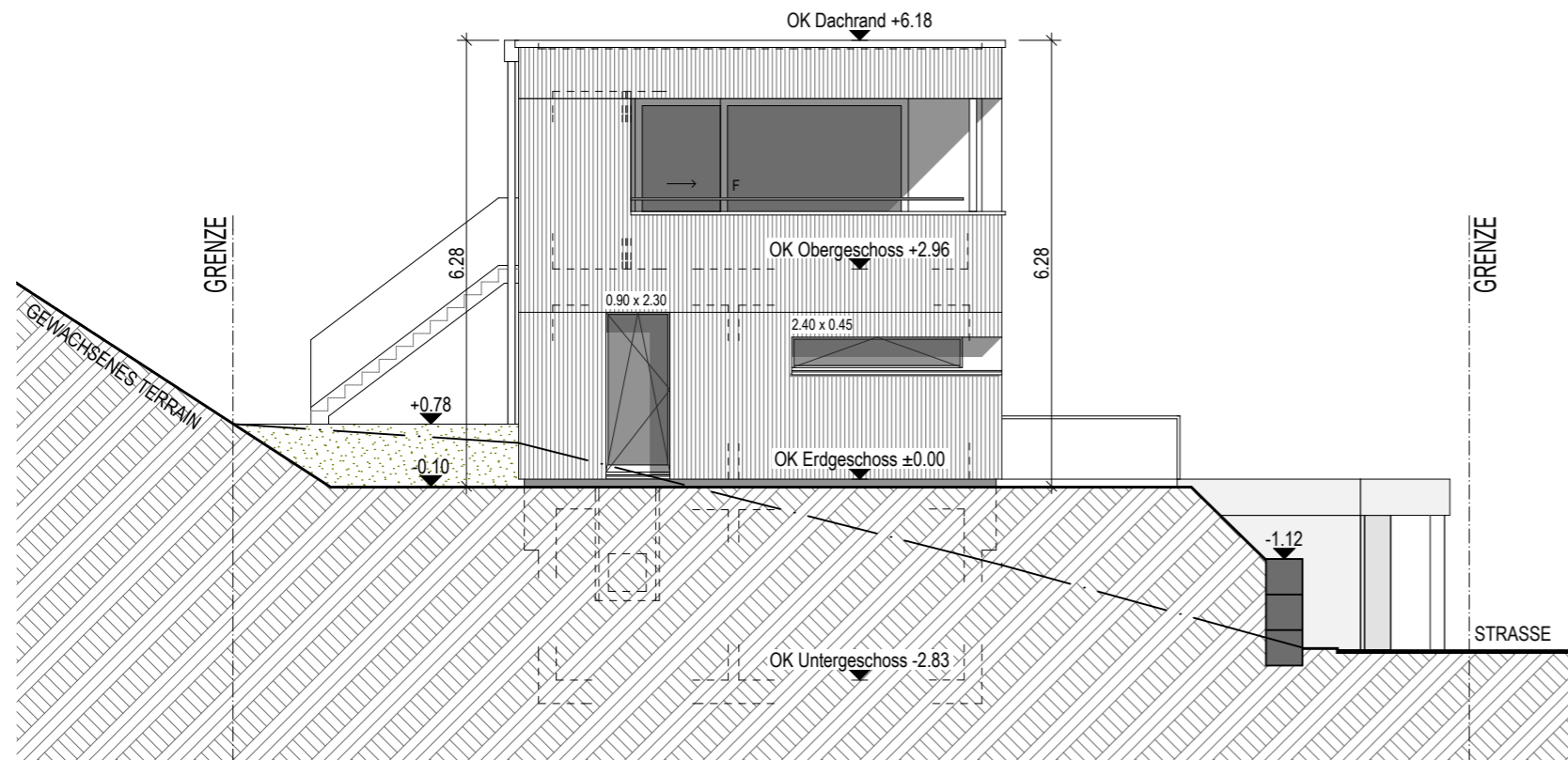
Ansicht Westen
