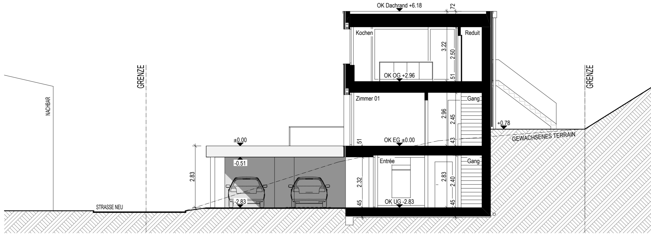
SCHNITT A
