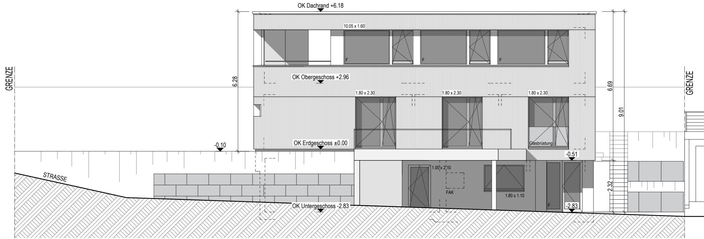
Ansicht Sueden
