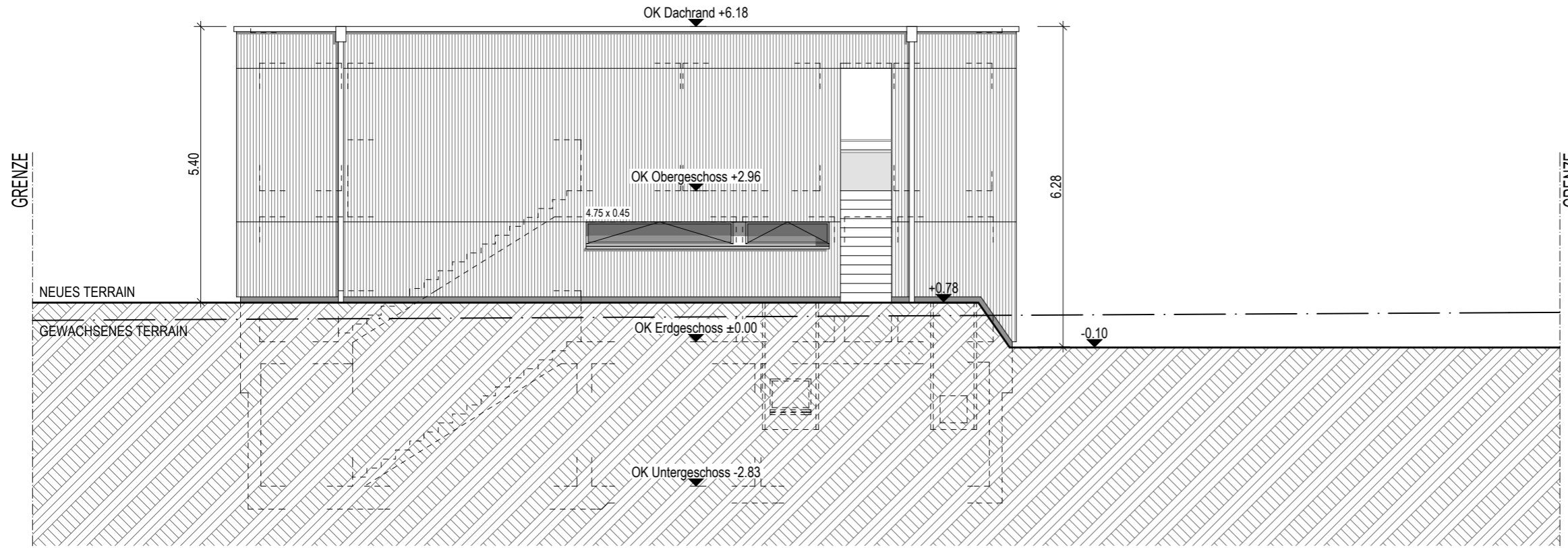
Ansicht Norden
