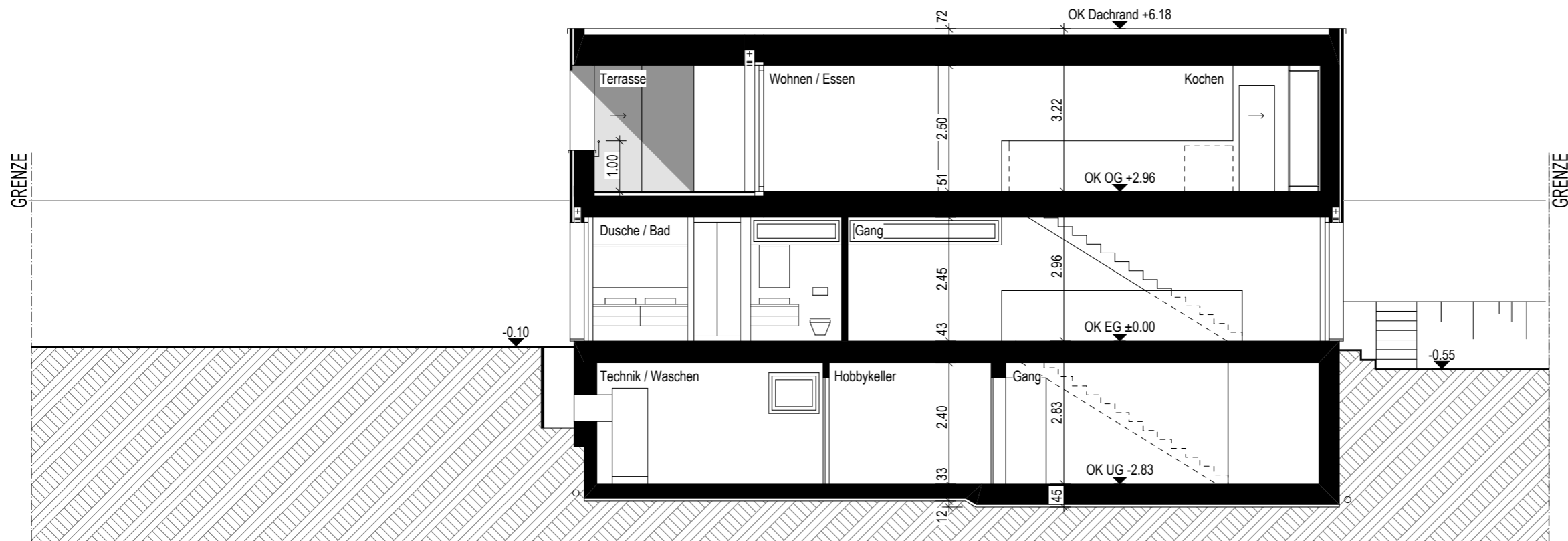
SCHNITT B
