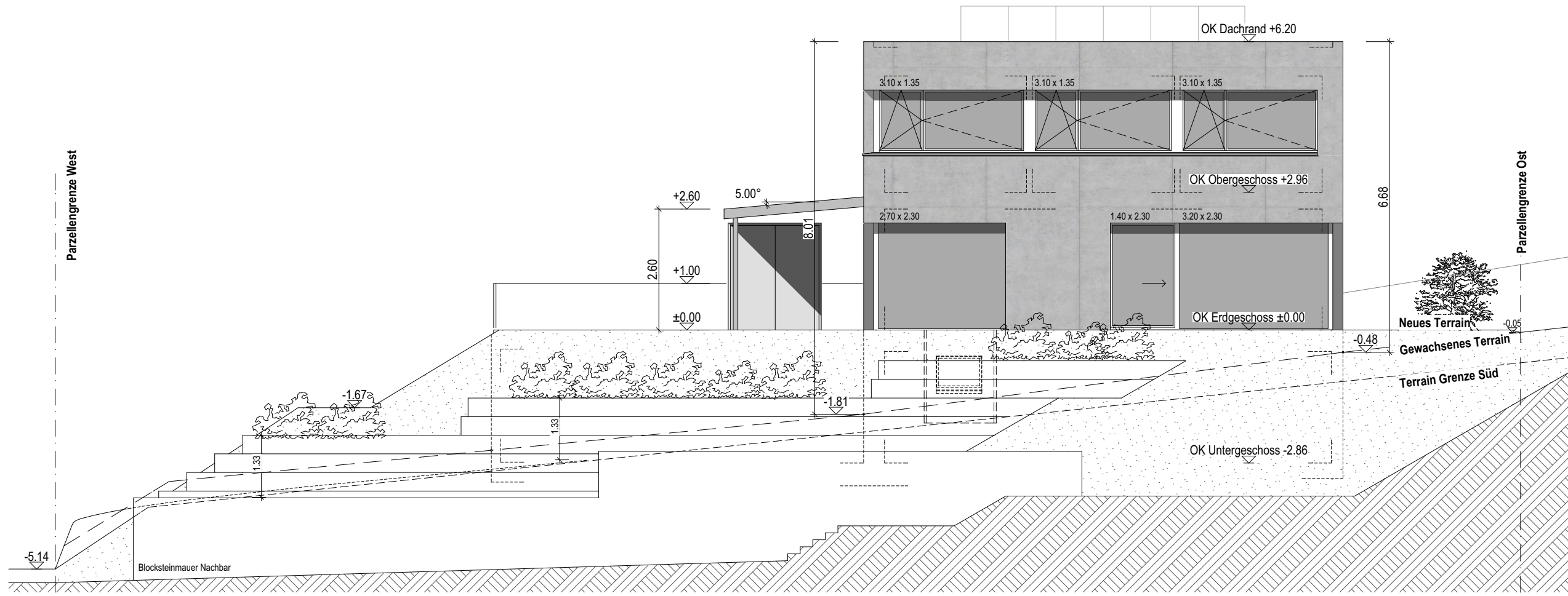
ANSICHT SUEDEN
