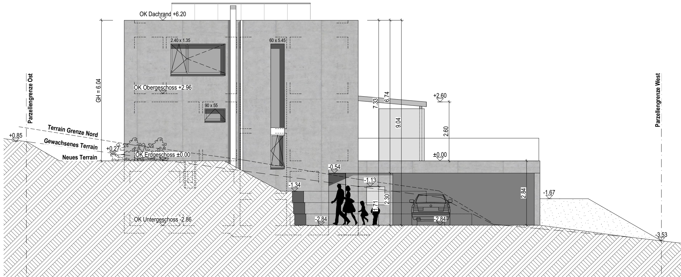
ANSICHT OSTEN
