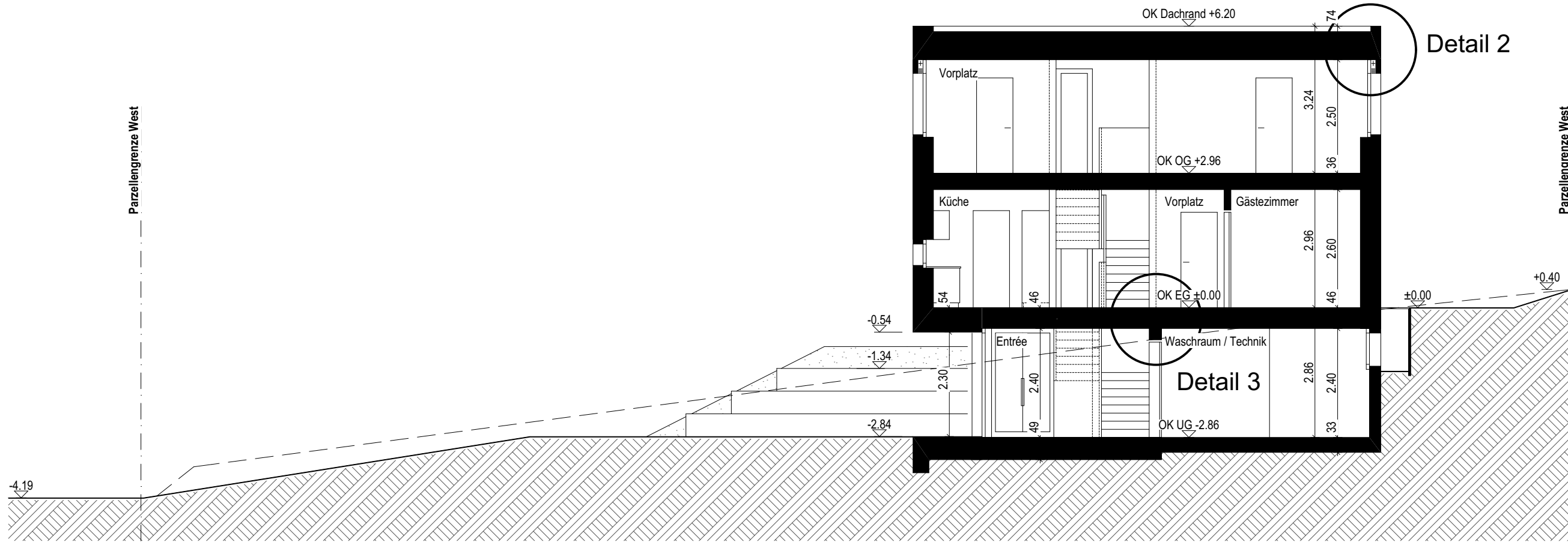
SCHNITT A
