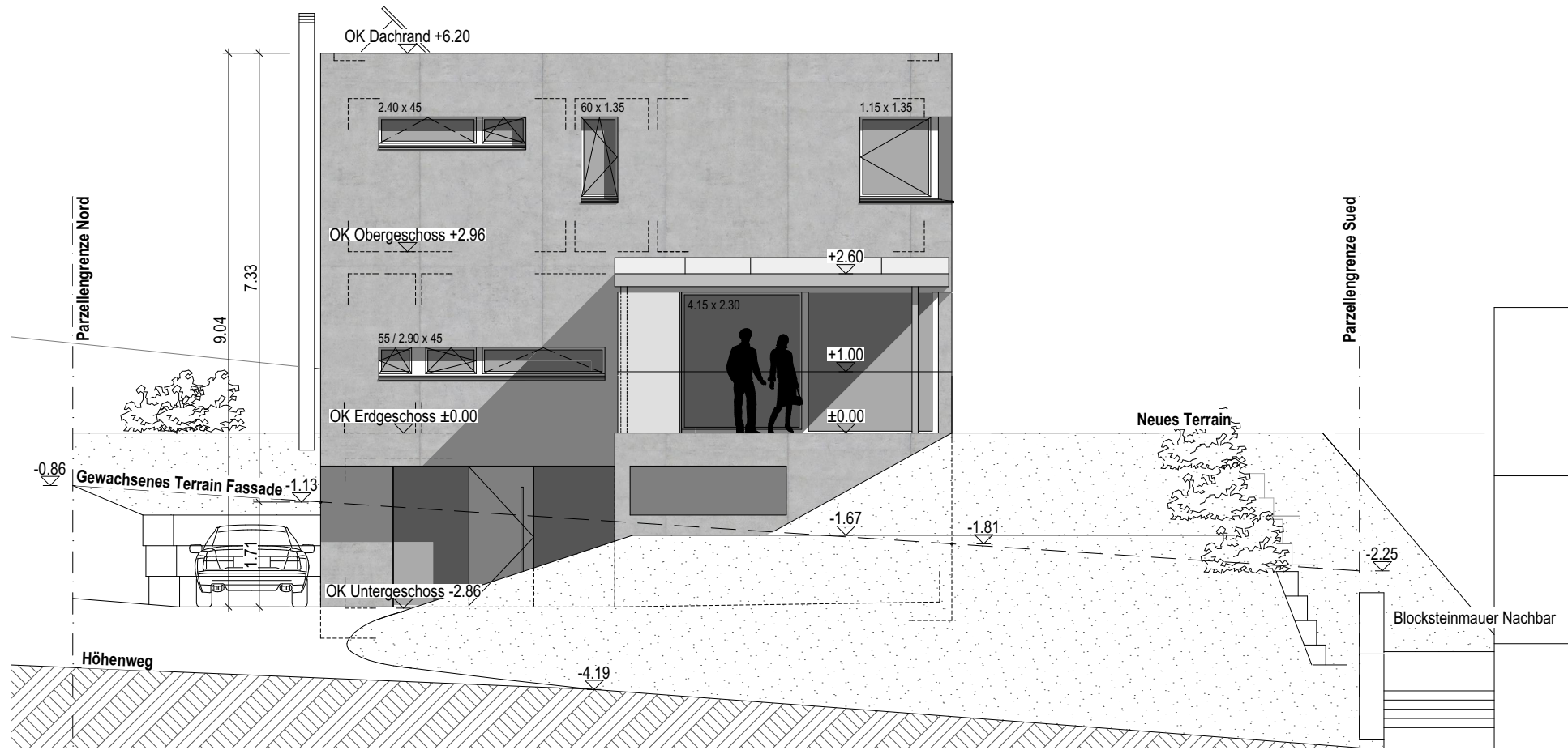
ANSICHT WESTEN
