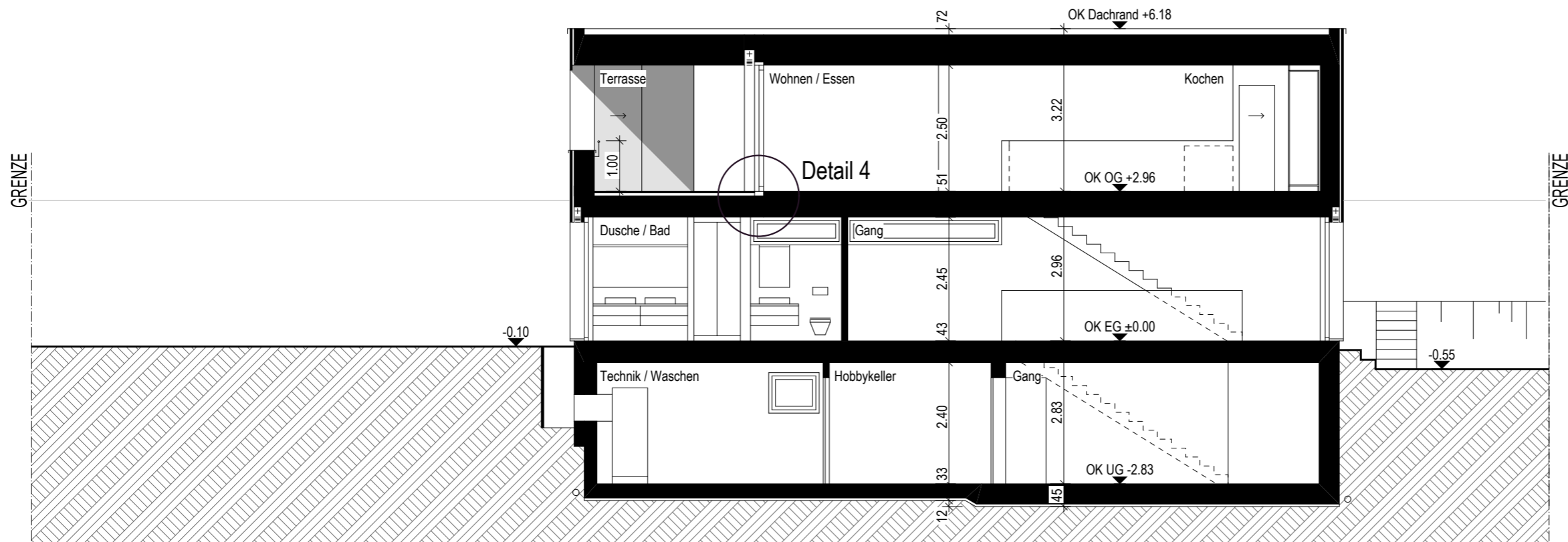
SCHNITT B
