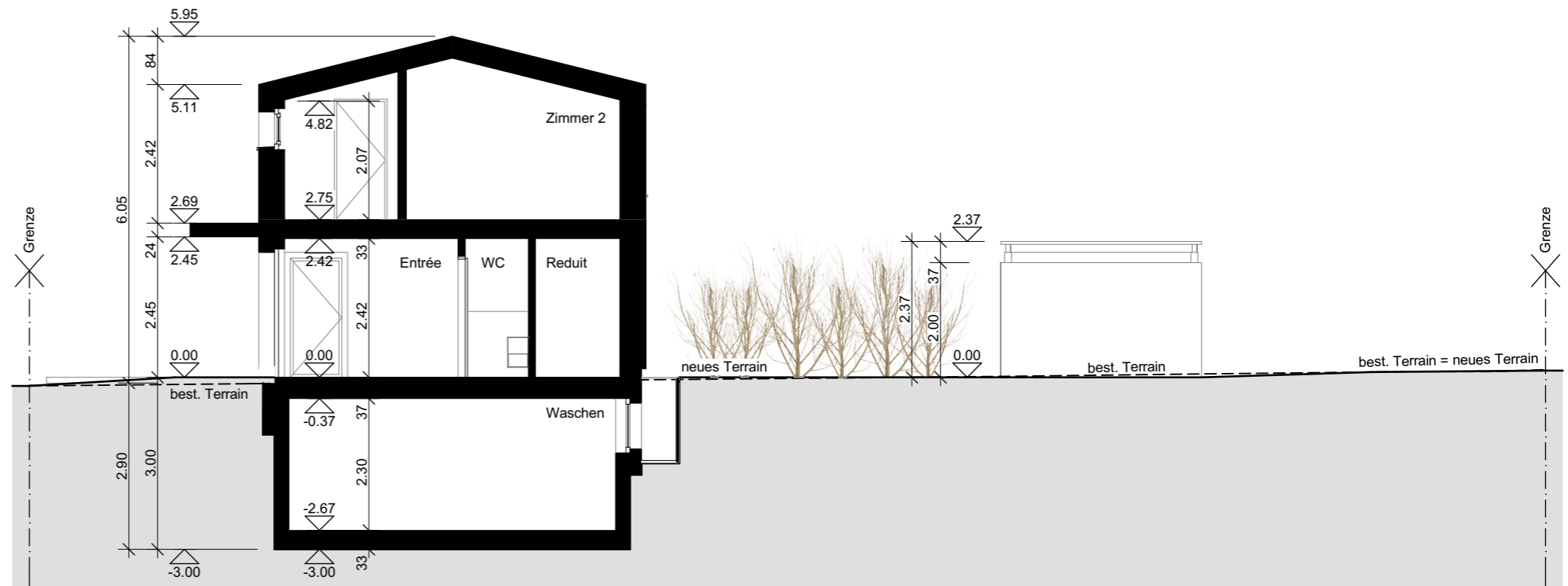
SCHNITT C
