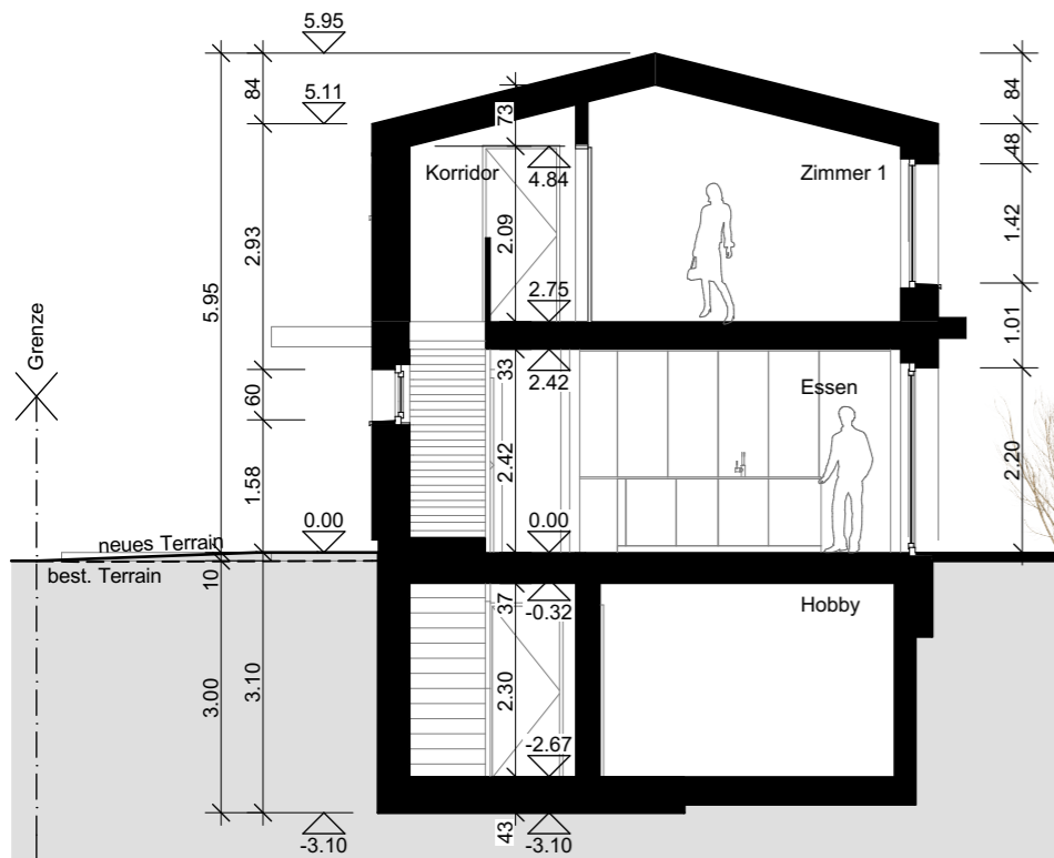
SCHNITT A
